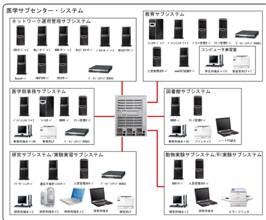
図 3.8: 医学サブセンターのシステム構成
