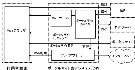
図 3 モジュール構成 Fig. 3 Module architecture.
