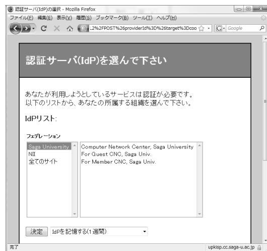
図 7 DS による IdP の選択
