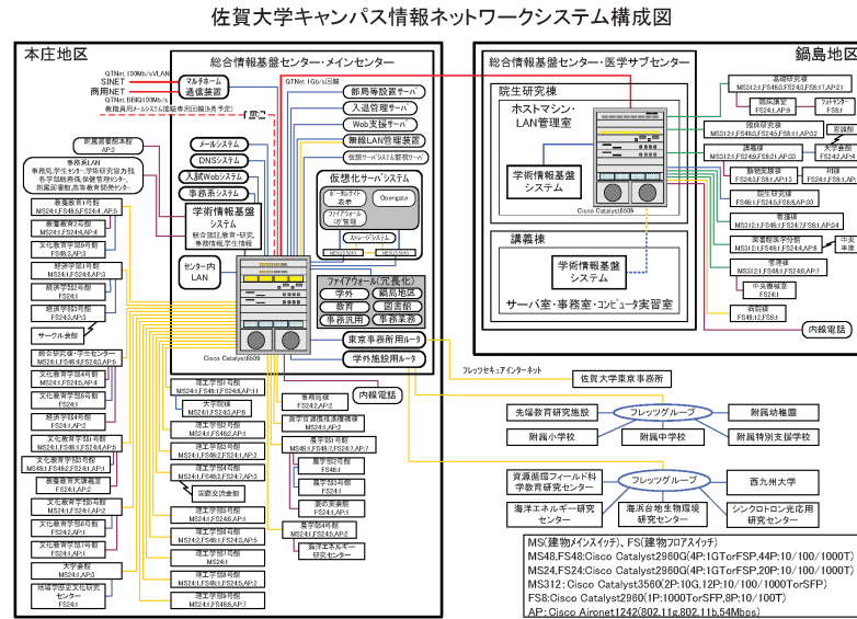
図 4.8: キャンパス情報ネットワークシステム構成
