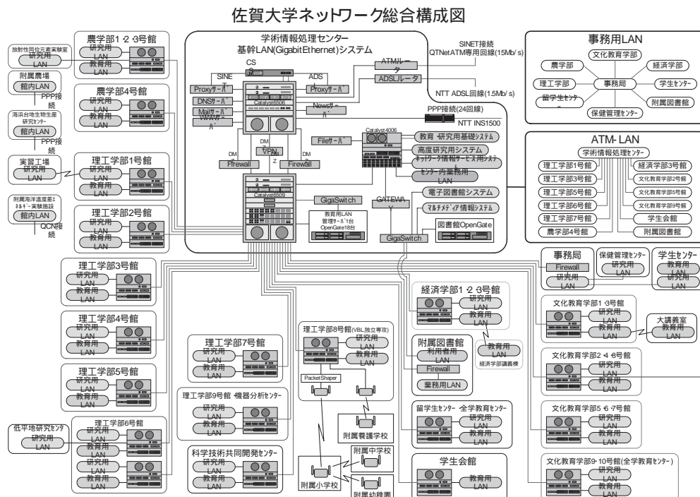
図 6.2: キャンパス情報ネットワークシステム構成
