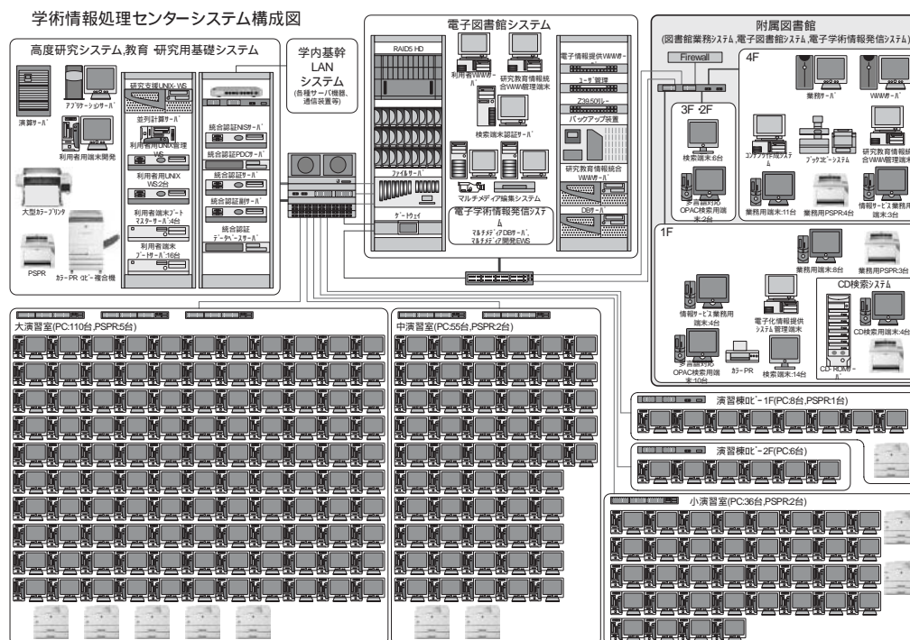
図 6.1: 学術情報処理センターのシステム構成
