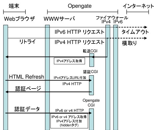
図 2 利用者端末のアドレス取得の流れ
